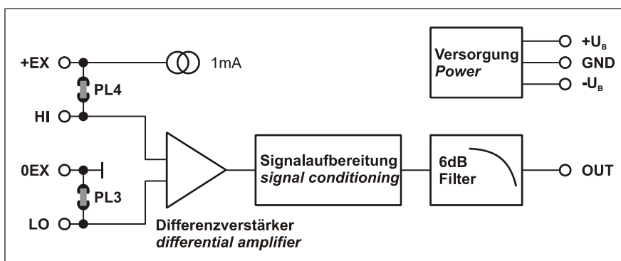
Funktionsschaltbild
