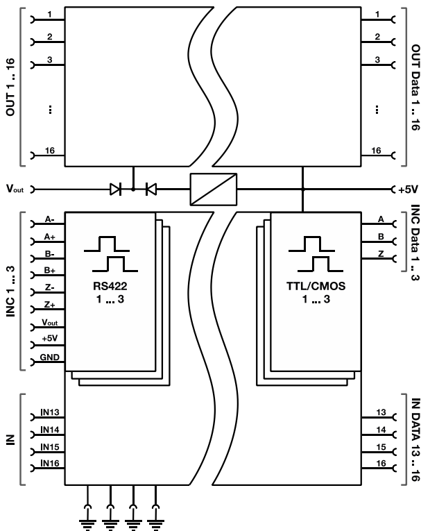
Funktionsschaltbild
