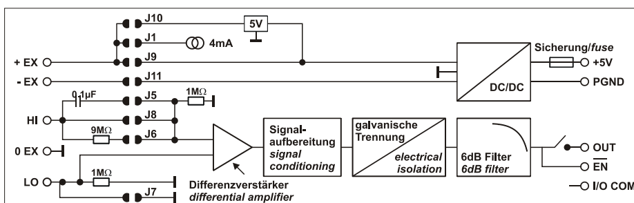
Funktionsschaltbild
