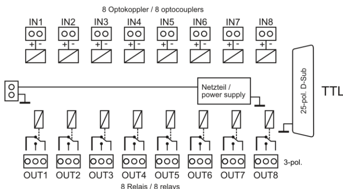
Funktionsschaltbild
