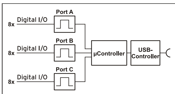
Funktionsschaltbild und Pinbelegung
